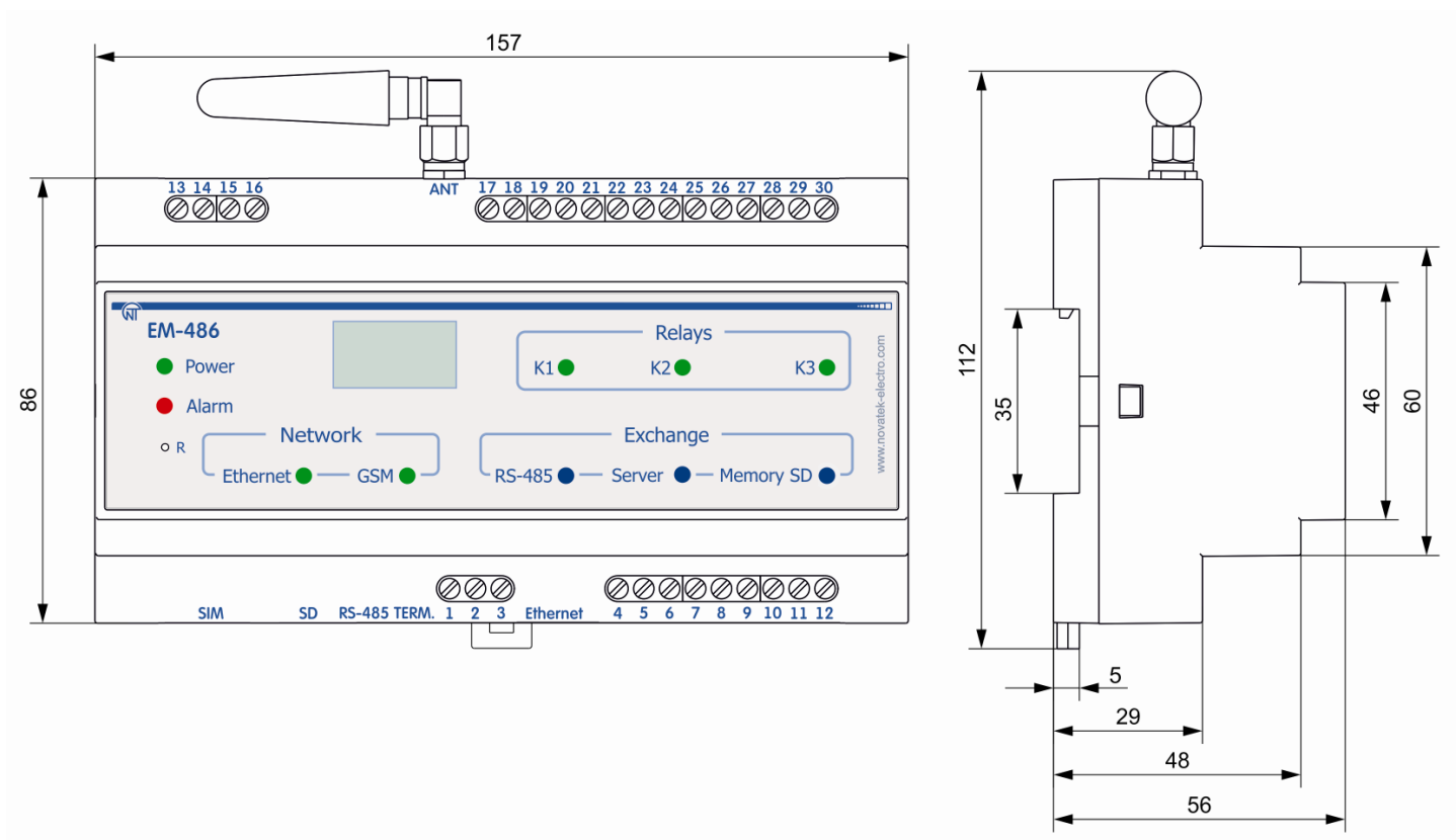
Рисунок 1.1 – Габаритні та установчі розміри EM-486
