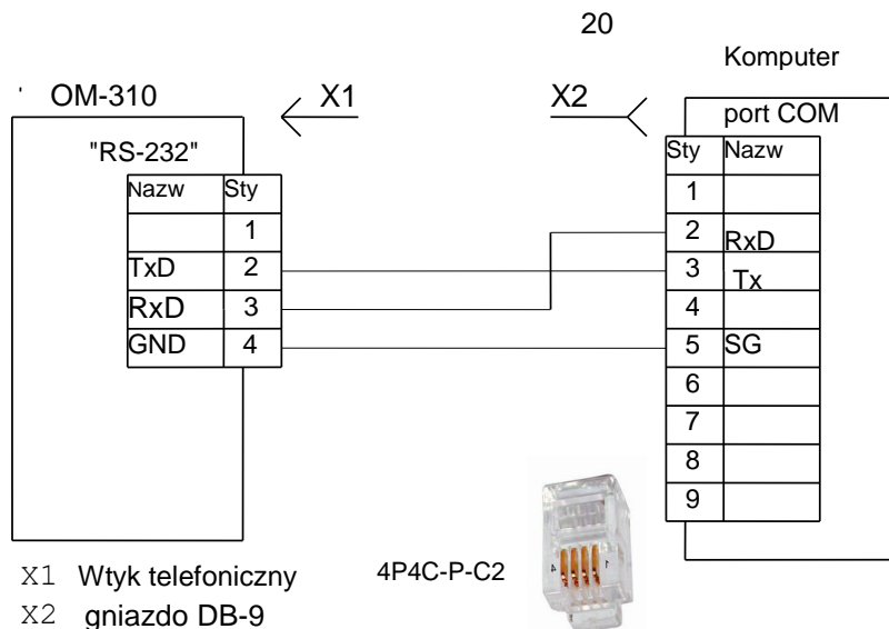
Rysunek 2.2. Schemat podłączenia OM-310 do komputera
