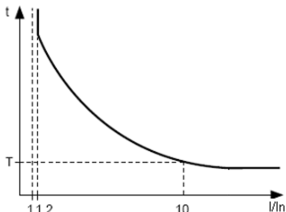
Rysunek 1.5. Zasada działania zabezpieczenia zwłocznego zależnego
