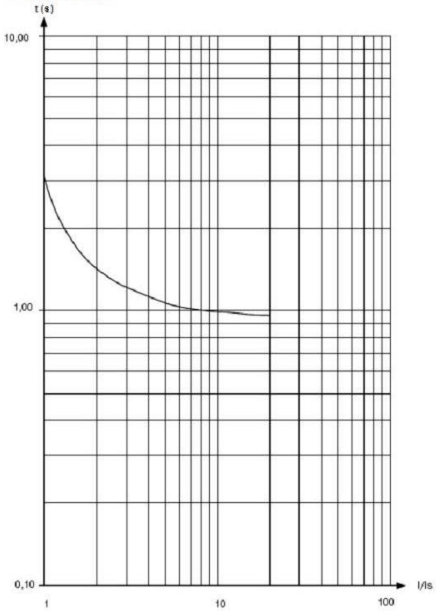
Krzywa zwłoki R1
