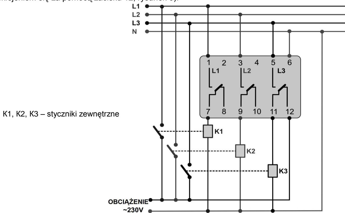
Rysunek 3 - Schemat podłączenia PEF-301 przy obciążeniu przekraczającym 16 A z wykorzystaniem elektromagnetycznych styczników zewnętrznych.
