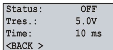
Rysunek 7.6.5. Ekran ustawienia górnego i dolnego progu zdarzenia
