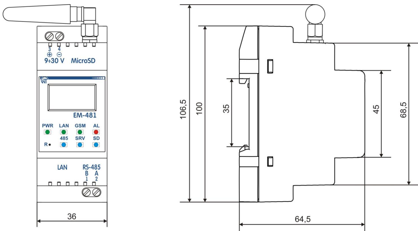
Рисунок 1.1 – Габаритні та установчі розміри EM-481
