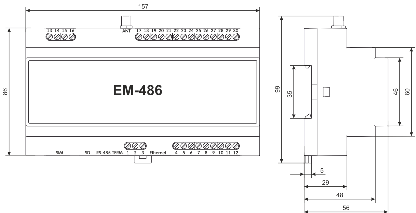
Рисунок 1.1 – Габаритні та установчі розміри ЕМ-486
