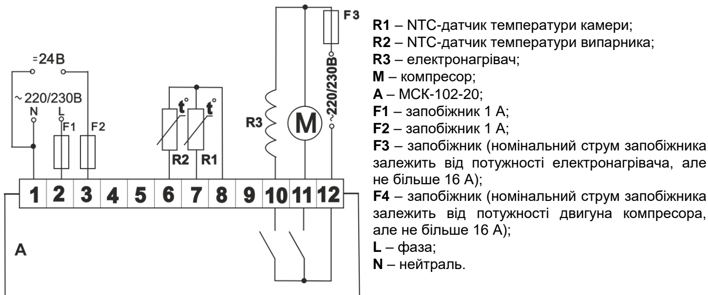
Рисунок 2 – Схема підключення МСК-102-20 до електричної мережі.
