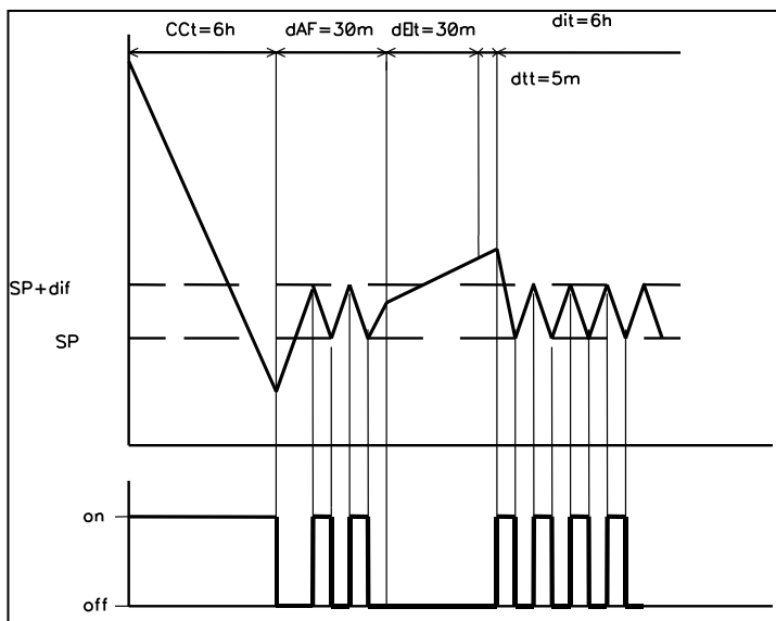
Рисунок 4 – Графік роботи МСК-102-20 в режимі «Набір холоду»
