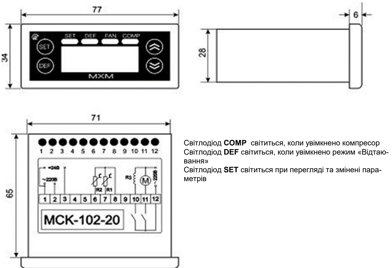
Рисунок 1 - Органи управління та габаритні розміри МСК-102-20
