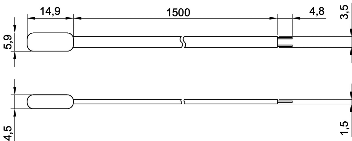
Рисунок 2 - Внешний вид и габаритные размеры
