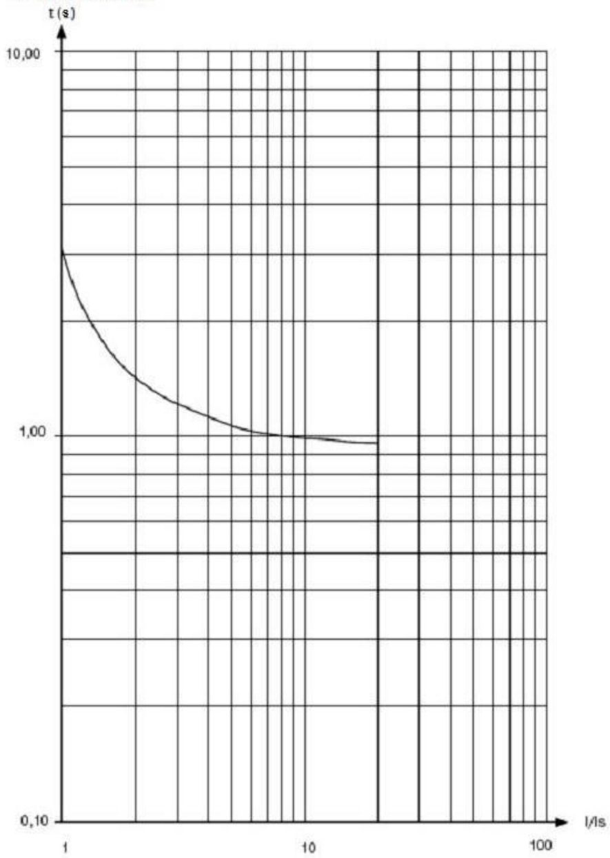
Krzywa zwłoki R1
