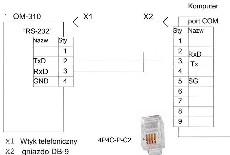
Rysunek 2.2. Schemat podłączenia OM-310 do komputera
