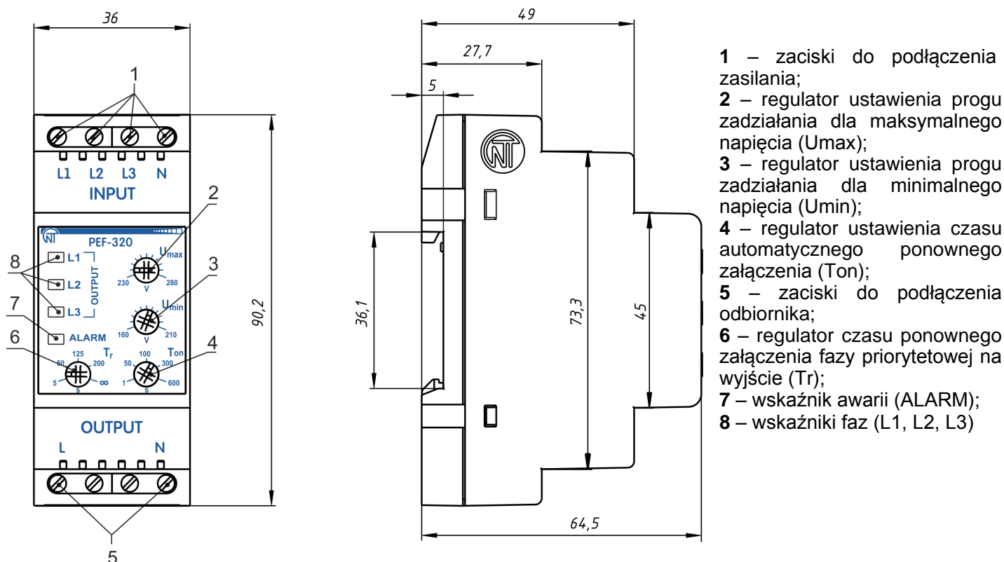
Rysunek 1. Organy sterujące, wymiary gabarytowe i montażowe
