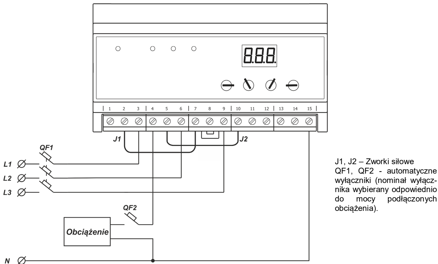
Rysunek 2. Schemat podłączenia PEF-319 przy obciążeniu nie przekraczającym 30 A
