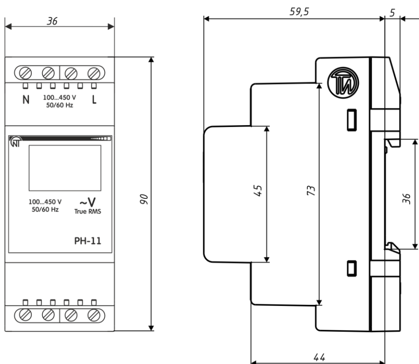
Rysunek 1. Wymiary gabarytowe i montażowe PH-11
