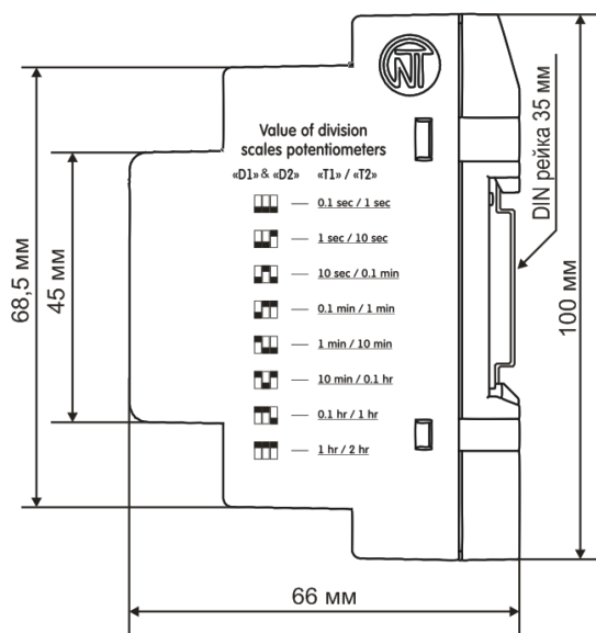
Рисунок 1 - Зовнішній вигляд і габаритні розміри
