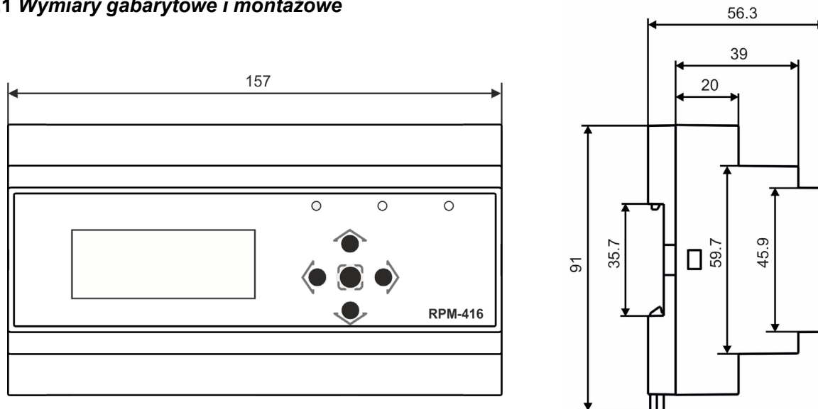
Rysunek 1.1. Wygląd zewnętrzny i wymiary gabarytowe rejestratora
