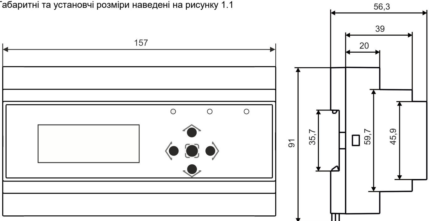
Рисунок 1.1 – Габаритні і установчі розміри реєстратора
