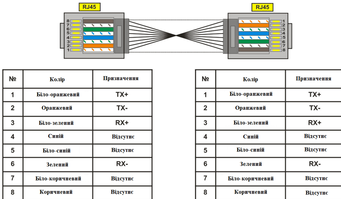
Рисунок 5.3 – Нумерація виводів кабелю з'єднання з мережею Ethernet
