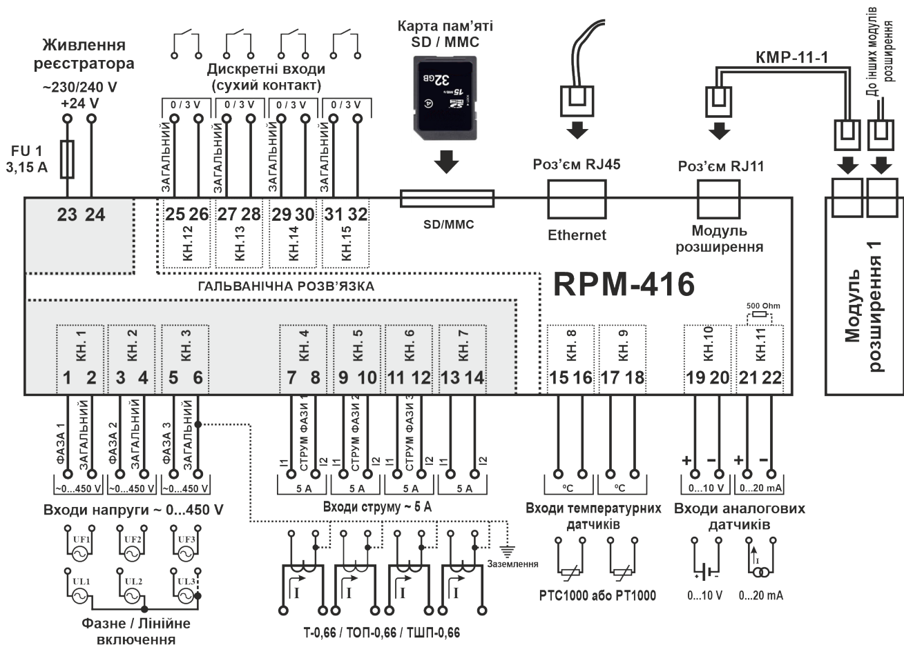
Рисунок 5.1 – Схема підключення RPM-416
