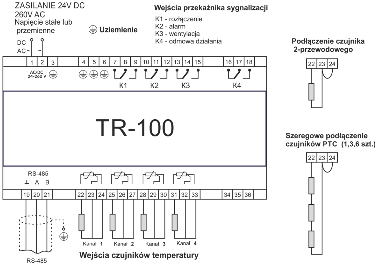
Rysunek 2 - Połączenia elektryczne TR-100
