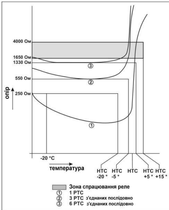
Рисунок 3 - Графік залежності опору від температури PTC датчиків
