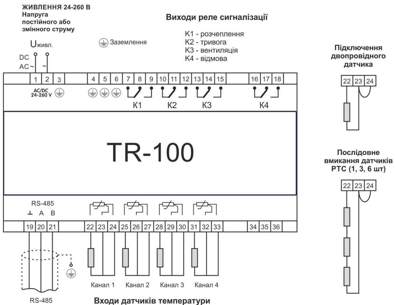
Рисунок 2 - Електричні з'єднання TR-100
