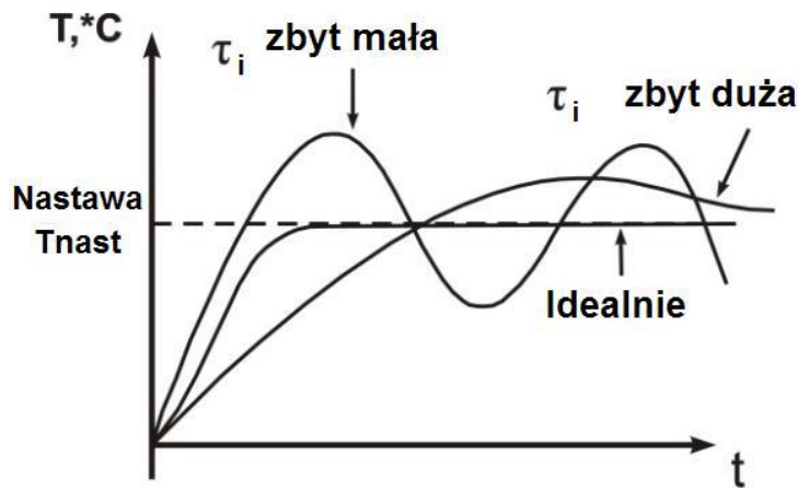
Rysunek 3.9 - Wykres pracy regulatora całkującego
