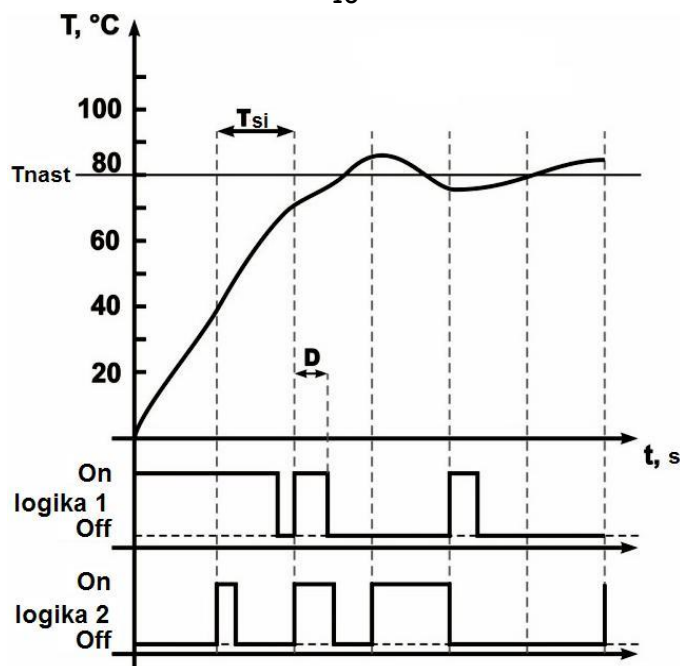
Rysunek 3.11 - Diagram zadziałania przekaźników wyjściowych w trybie regulacji PID
