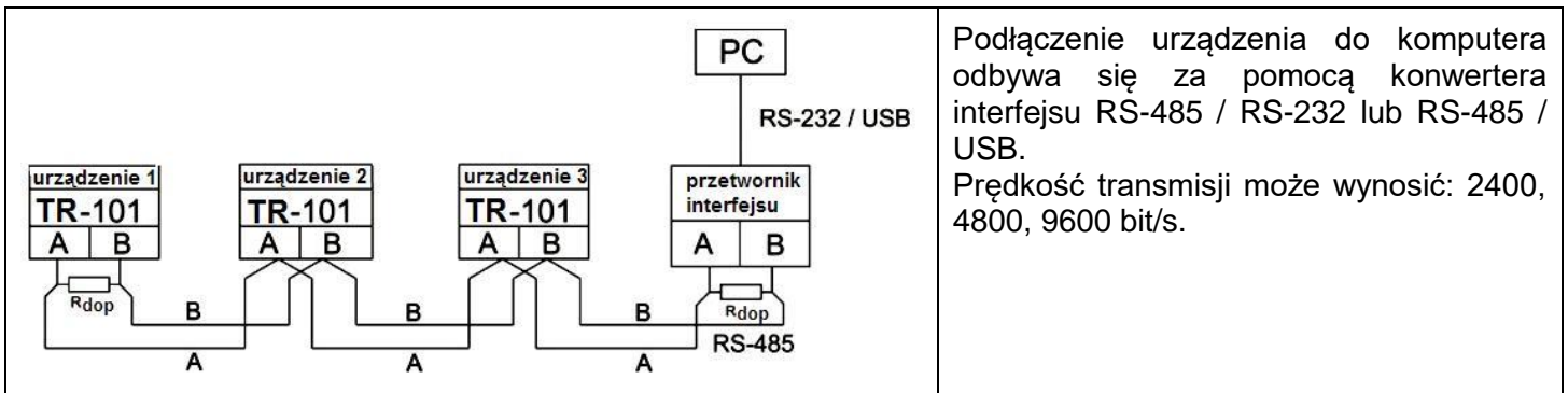
Rysunek A1 - Podłączenie urządzeń do sieci RS-485
