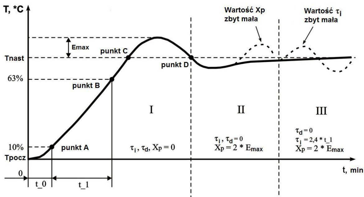
Rysunek 7.1 - Ręczne ustawienie regulatora PID
