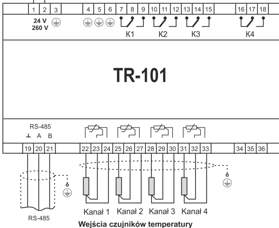
Rysunek 5.1 – Schemat podłączenia TR-101
