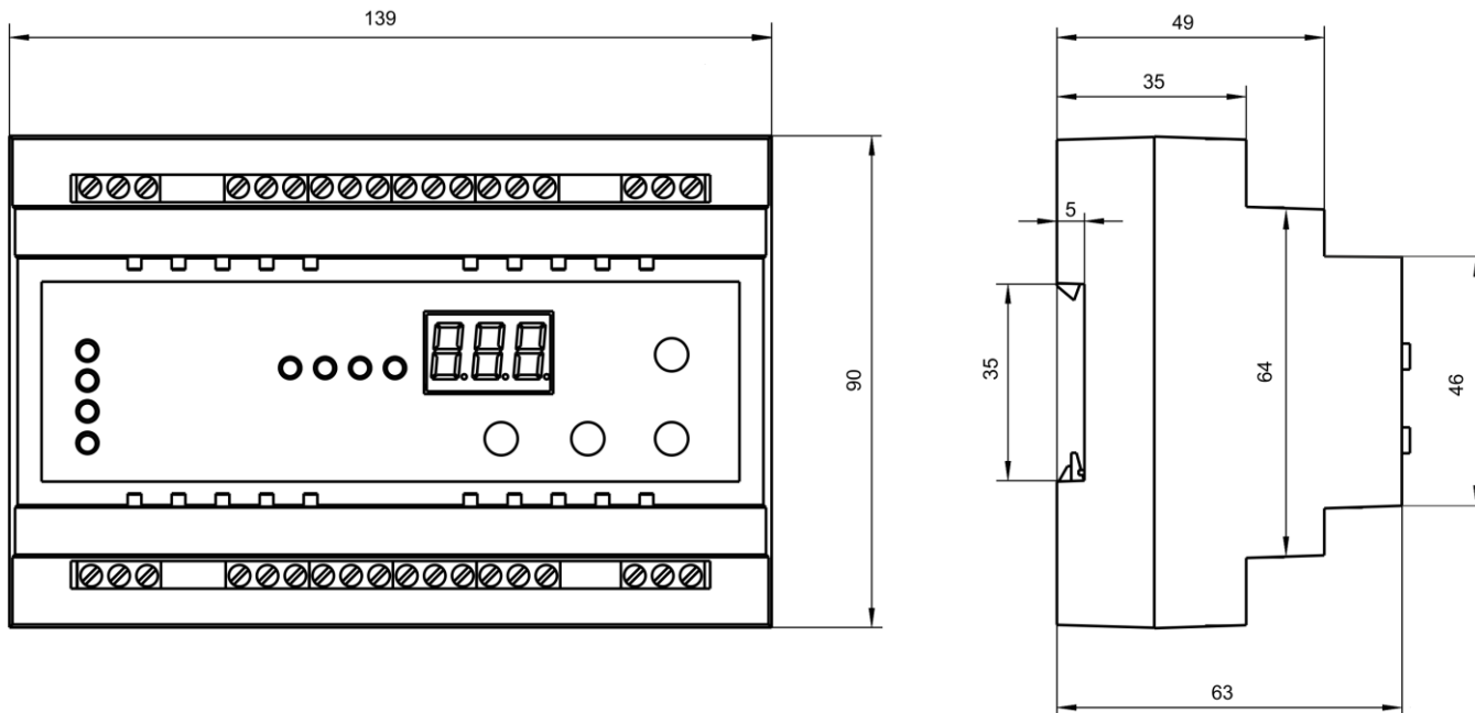
Rysunek 3.1 – Wymiary gabarytowe TR-101
