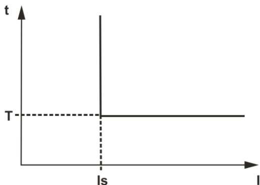
Rysunek 1.2 - Zasada działania zabezpieczenia zwłocznego niezależnego
