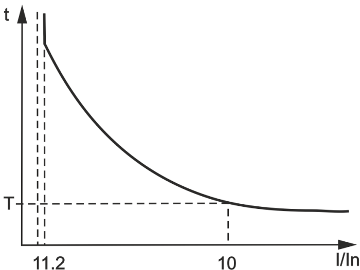
Rysunek 1.5 - Charakterystyka czasowo-prądowa
