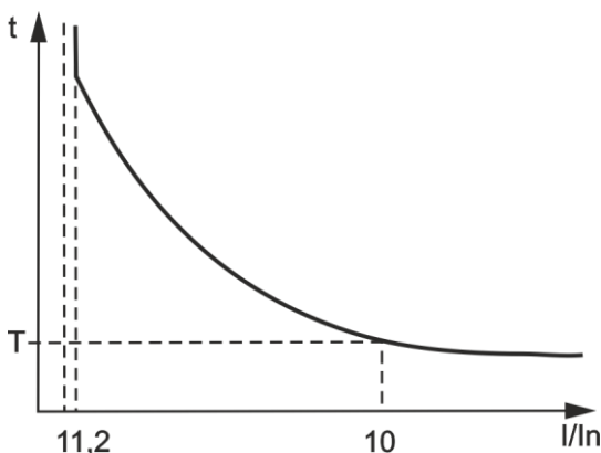
Rysunek 1.3 - Zasada działania zabezpieczenia zwłocznego zależnego
