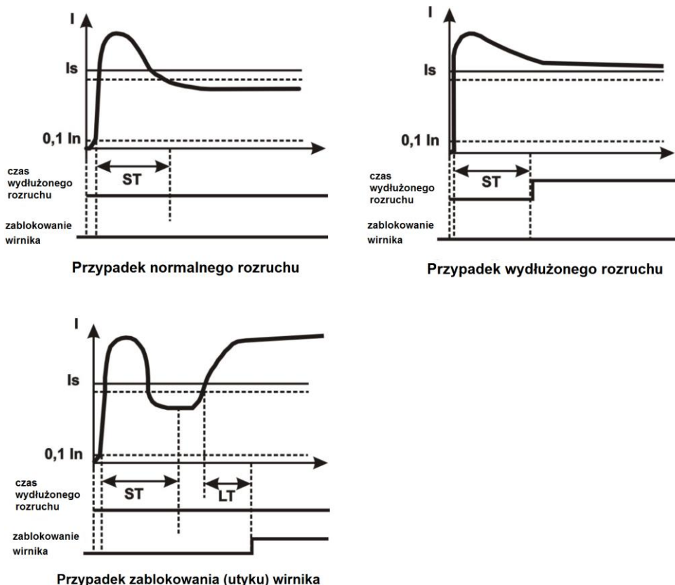
Rysunek 1.4 - Wydłużony rozruch i zablokowanie wirnika
